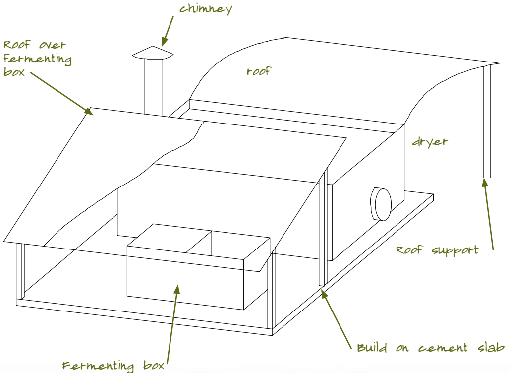
Mini dryer
